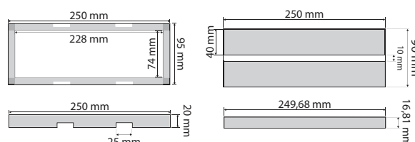
DIBUJO EN SECCIÓN REGISTROS OCULTOS
