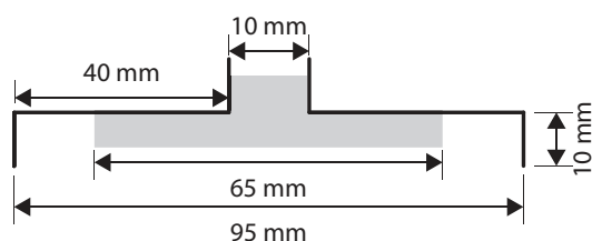
DIBUJO EN SECCIÓN REJILLAS OCULTAS
