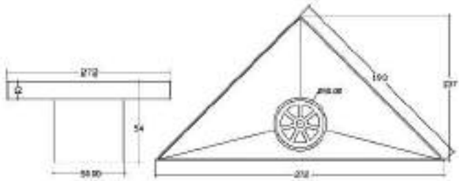
Llave extracción rejilla.
