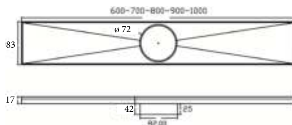
Llave extracción rejilla.
