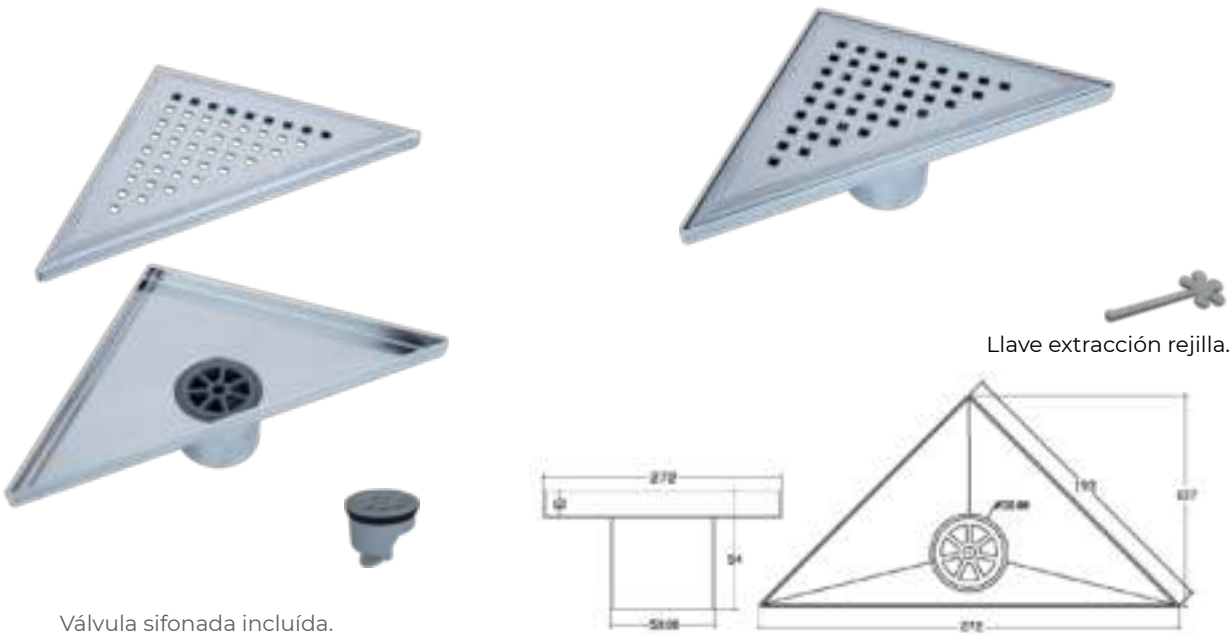
Válvula sifonada incluida.
